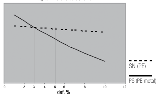
Force / deflection diagram Diagramme effort / déflexion
